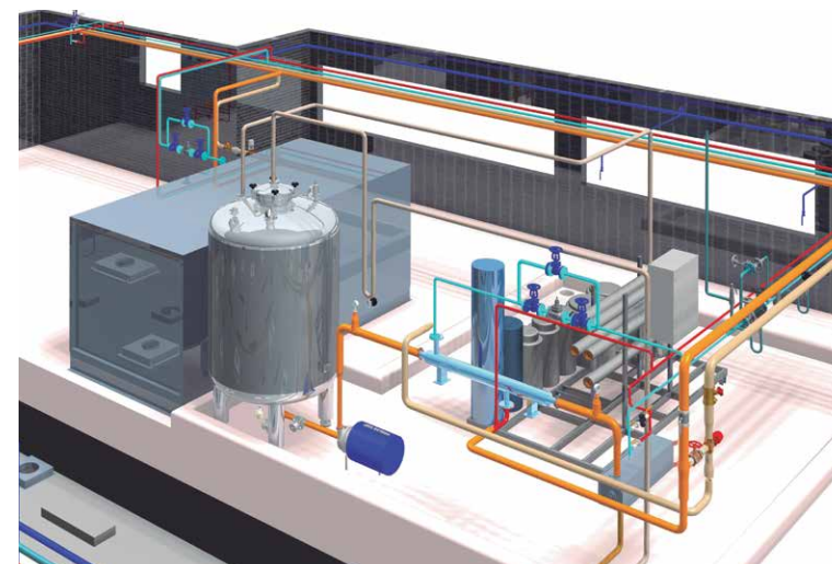
Génération et distribution d'eau purifiée (PW)
