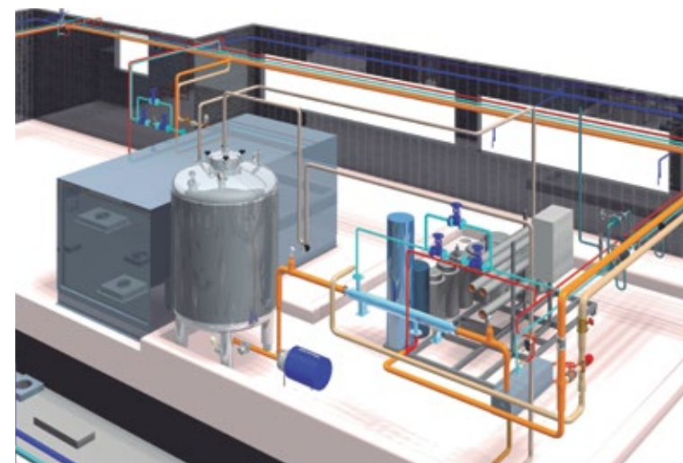
Generación y distribución de agua purificada (PW)
